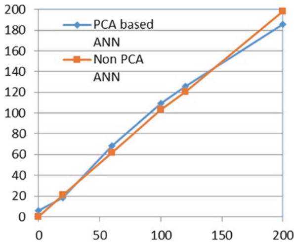
Fig. 17.7 ANN predictions
